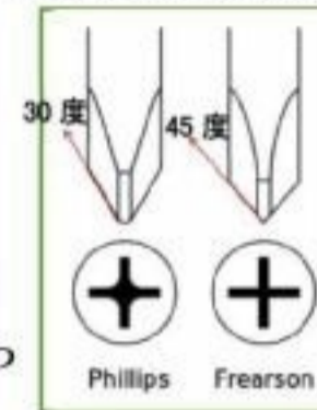
ネジの形とねじ回しの種類
